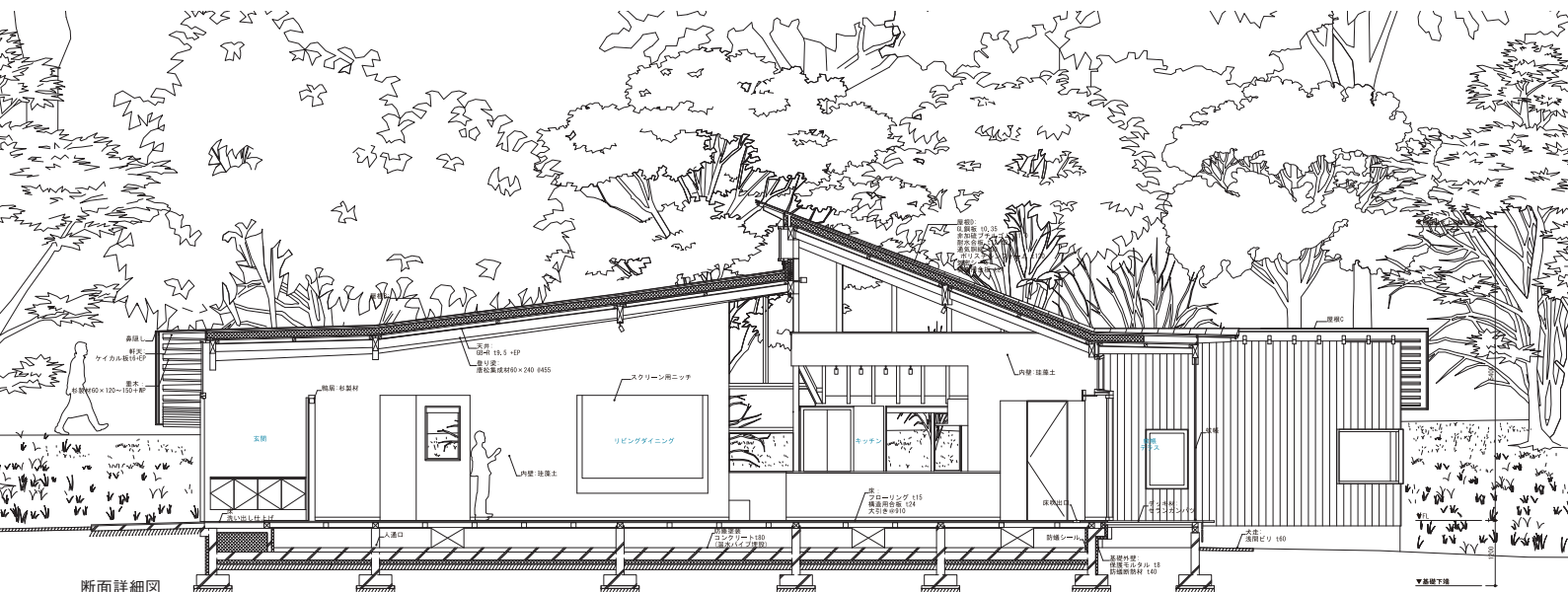
断面詳細図
